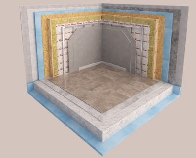
Entramado de Madera Ejecución de la vivienda en 11 meses
