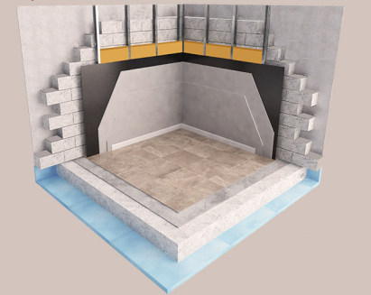
Bloque Hormigón Celular Ejecución de la vivienda en 13 meses
