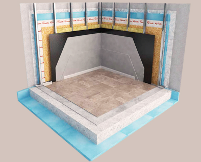
Entramado de Acero Ejecución de la vivienda en 11 meses
