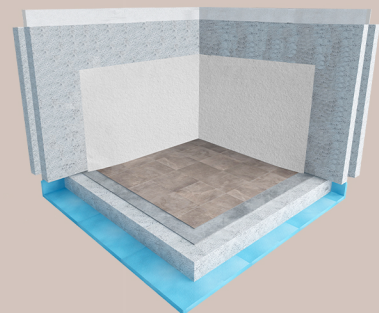
Hormigón 3D doble Ejecución de la vivienda en 9 meses
