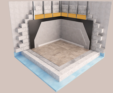
Bloque Hormigón Celular Ejecución de la vivienda en 14 meses
